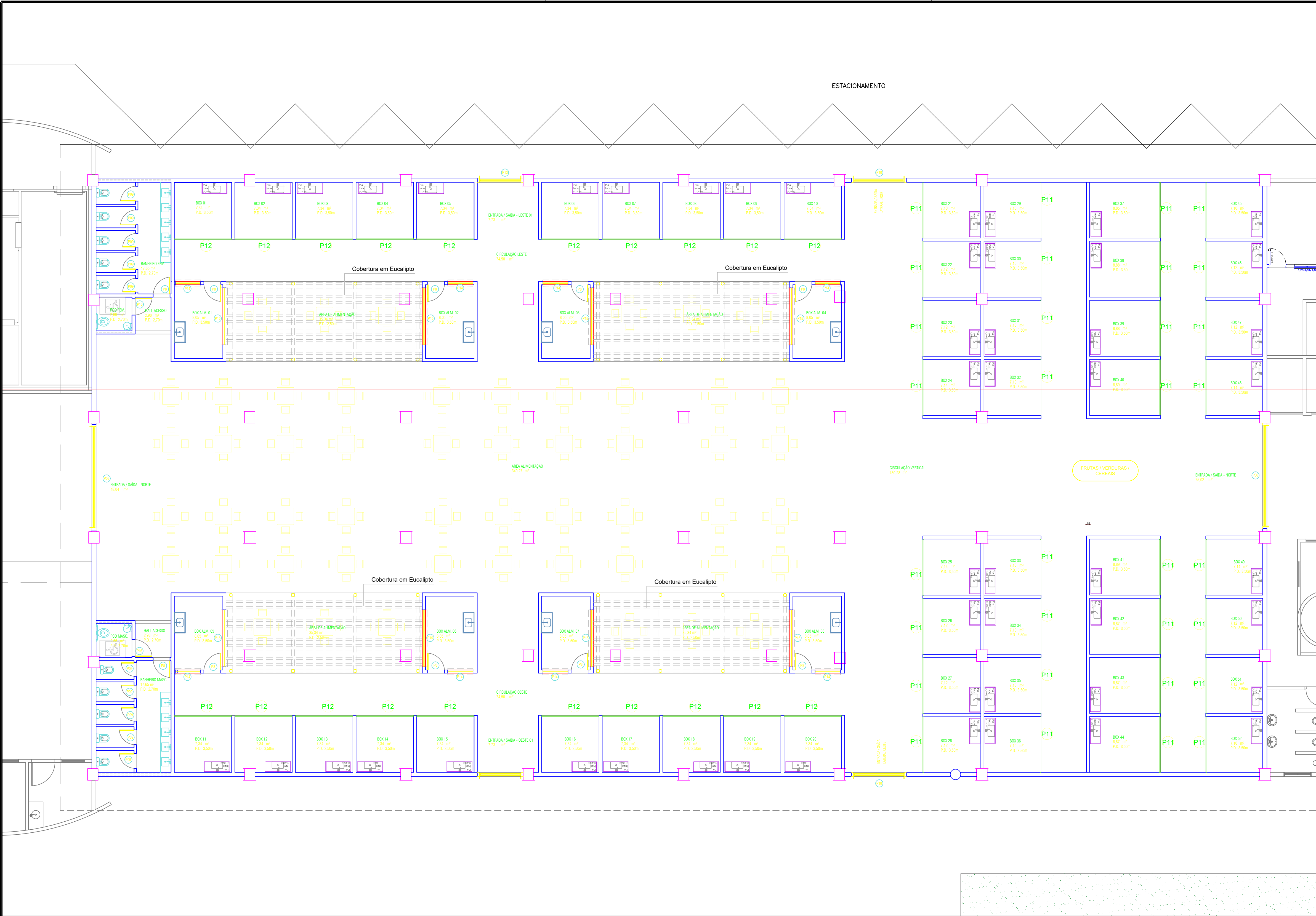
PLANTA DE LAY OUT esc. 1:150
