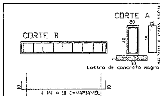
Figura 07: Detalhamento de Cinta de Confinamento
