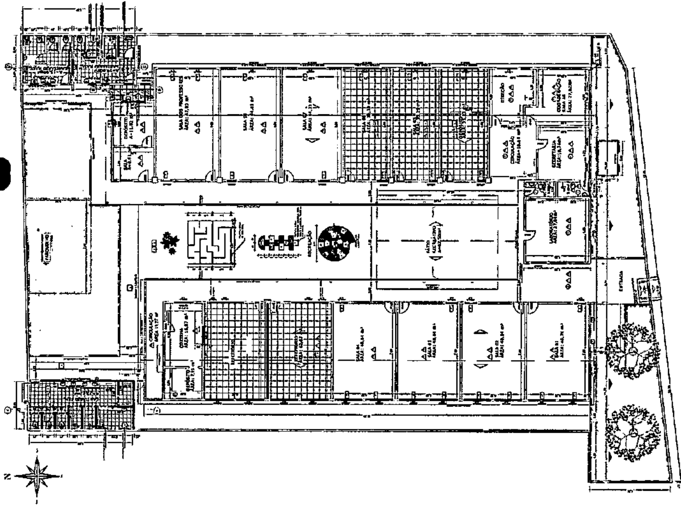
PLANTA BAIXA ESC. 1/150
